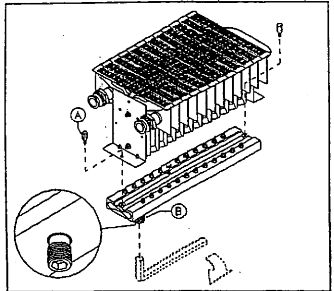
BRENNEREXPLOSIONSZEICHNUNG
