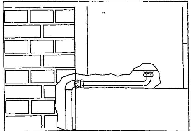
ROHRANSCHLUSSBEISPIEL
