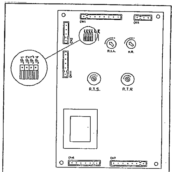
STEUERPLATINE
