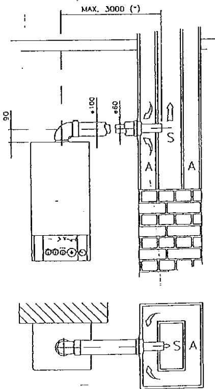
DOPPELROHR HORIZONTAL ZULUFT- UND ABGASFÜHRUNG IN KAMIN
