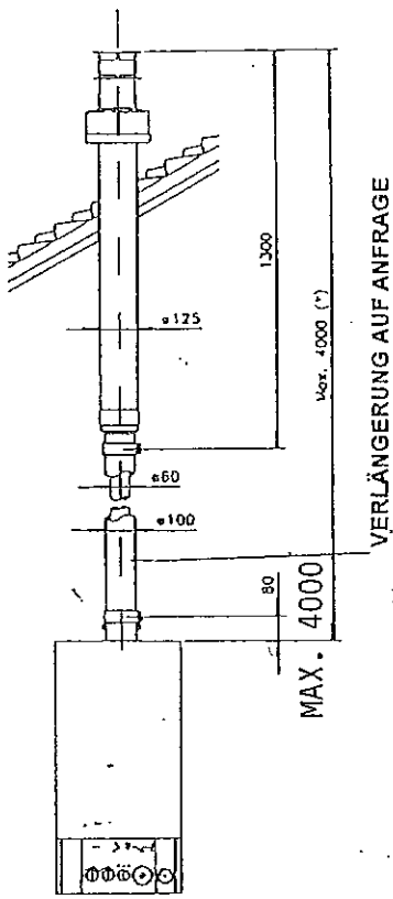
SENKRECHTES DOPPELROHR KIT
