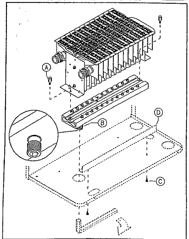
BRENNEREXPLOSIONSZEICHNUNG
