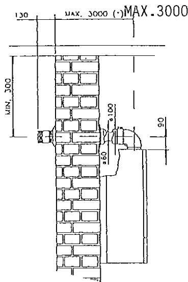
DOPPELROHR HORIZONTAL KIT
