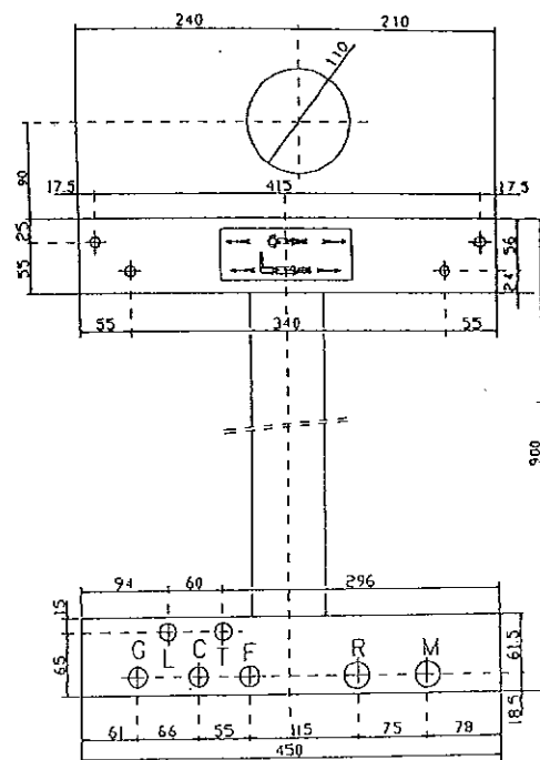
MONTAGESCHABLONE ECOLASER 20 SE
