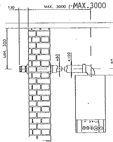
DOPPELROHR HORIZONTAL KIT
