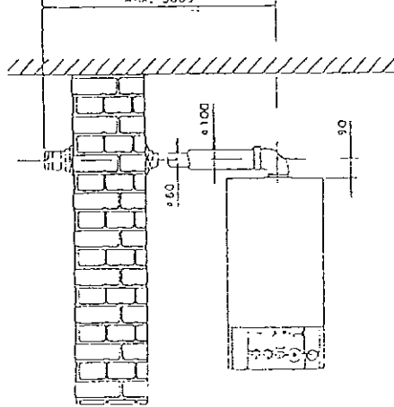
BEI GERADER ROHRFÜHRUNG MAX. 3000
